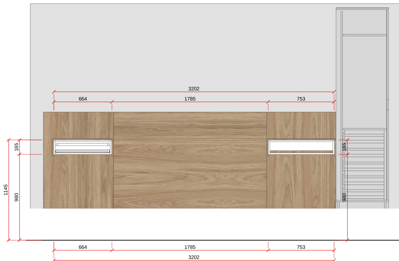
VISTA A - ESC. 1:25
